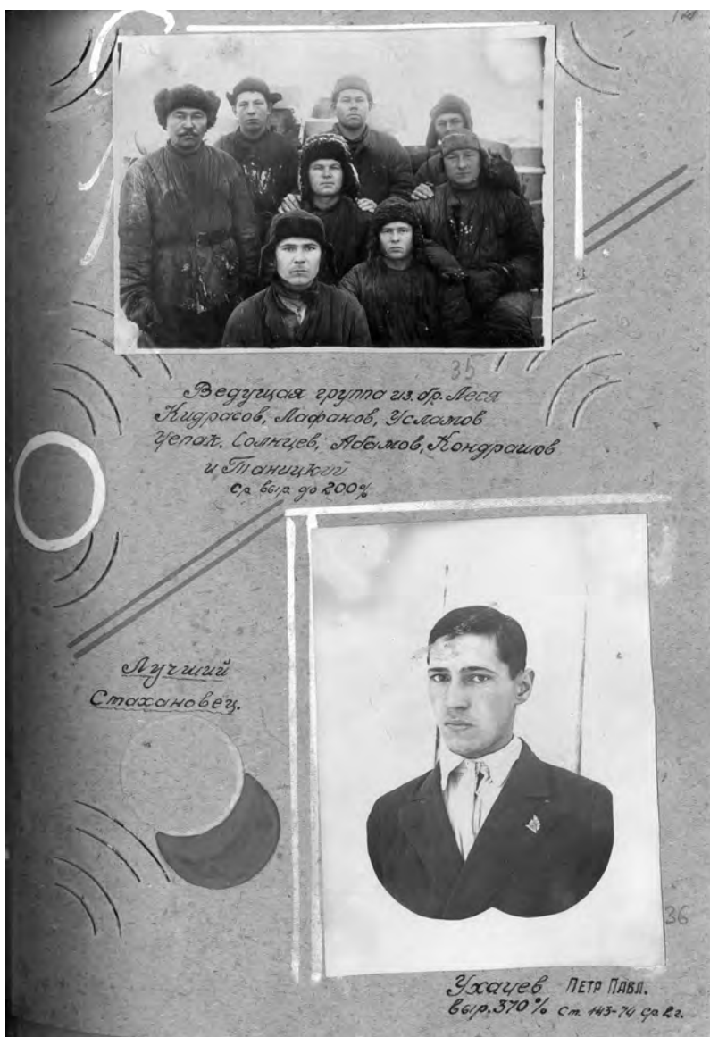
Рис. 7.2. Страница из фотоальбома «Стахановцы Девятого Управления ББК-НКВД», приблизительно 1934–1936 годы (Национальный архив Республики Карелия)
